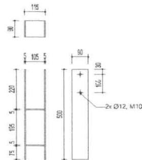
OCEĽOVÁ KOTVA
